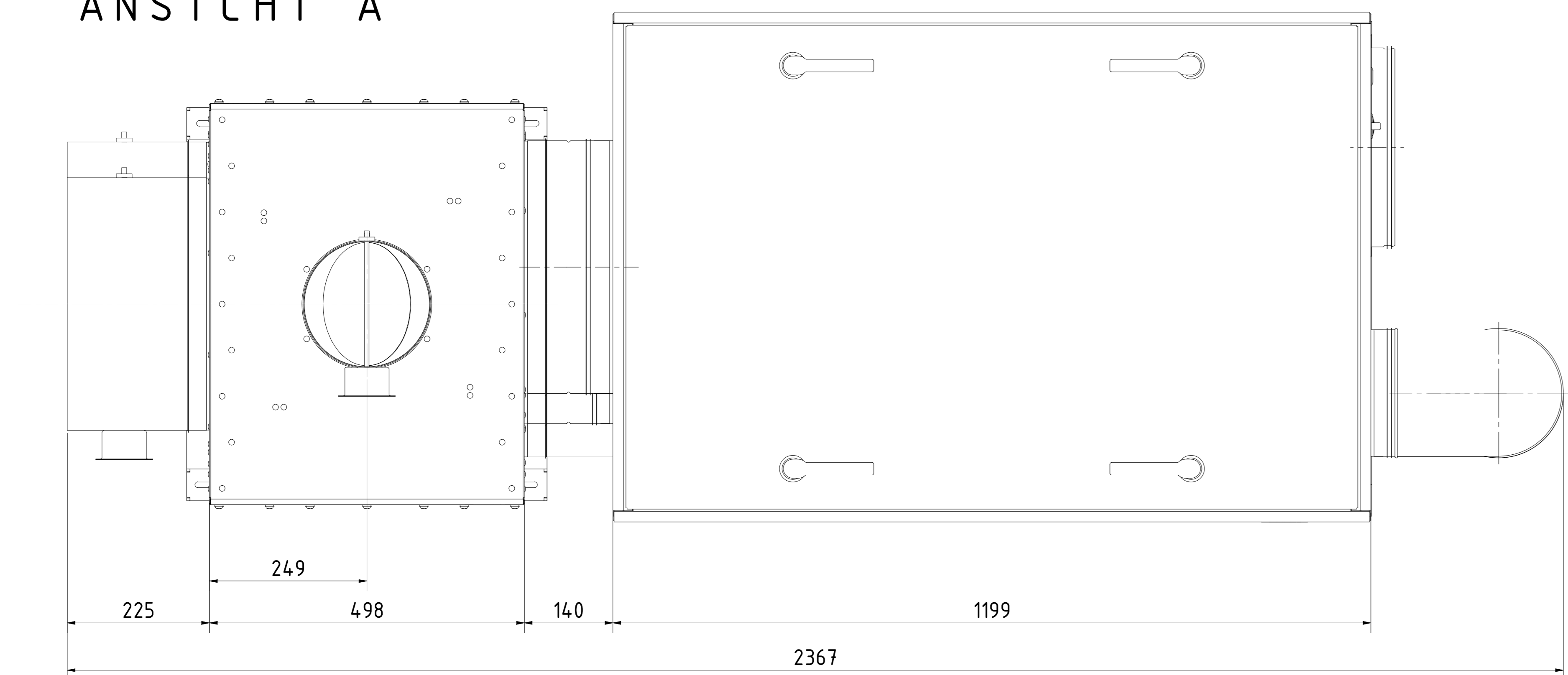
ANSICHT A
